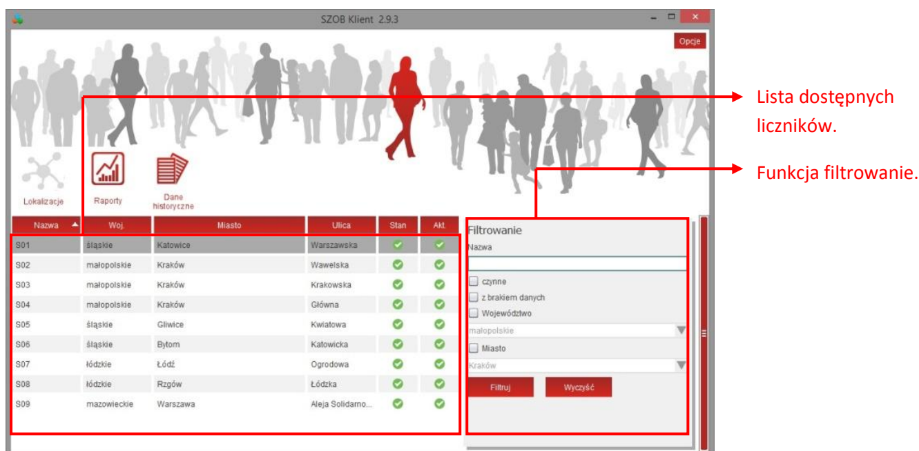
Okno lokalizacji.
